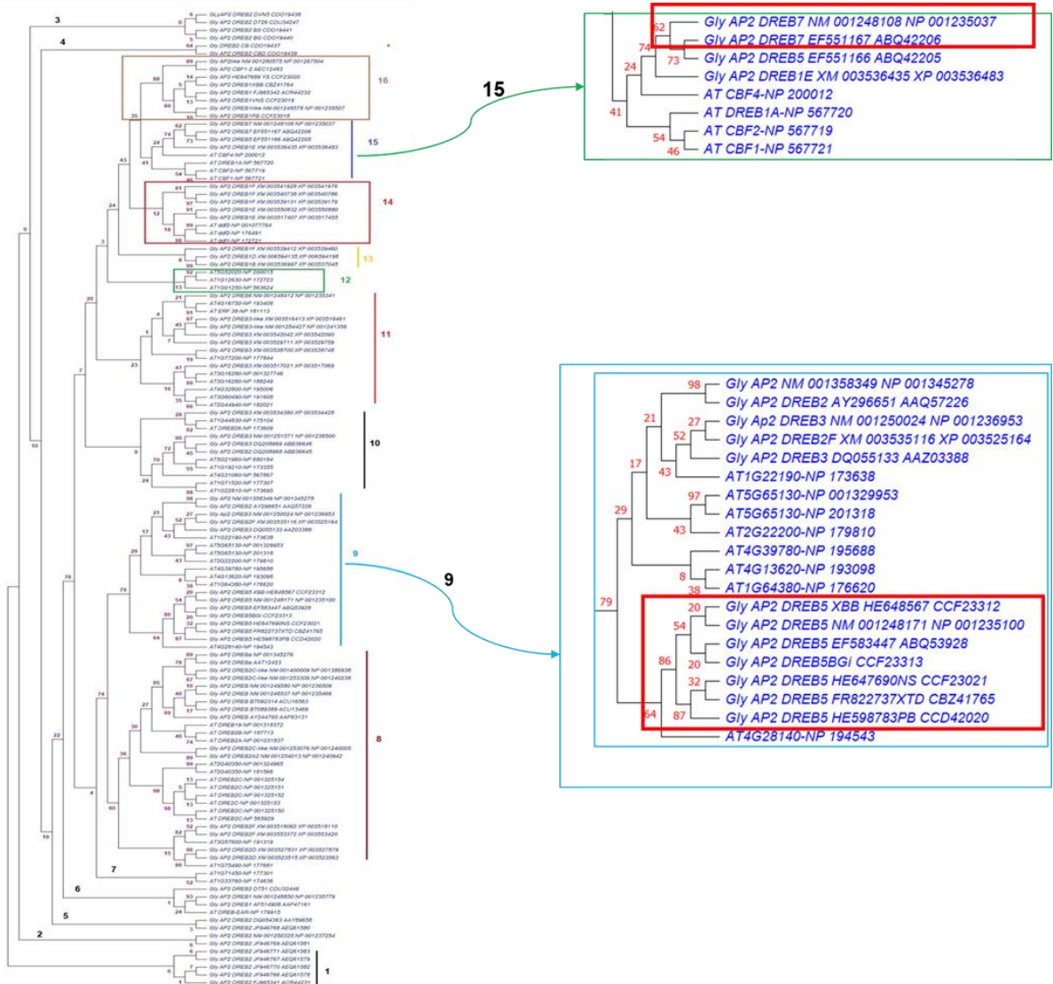
Hình 3.3. Sơ đồ phát sinh chủng loại miền AP2 của phân họ protein DREB5 và DREB7 ở cây A. thaliana và đậu tương theo phương pháp Maximum likelihood.
