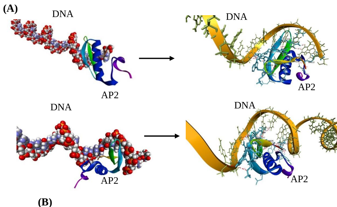
Hình 3.14. Mô hình liên kết AP2 - promoter và mạng lưới liên kết hydrogen (H) giữa AP2 và DNA.
