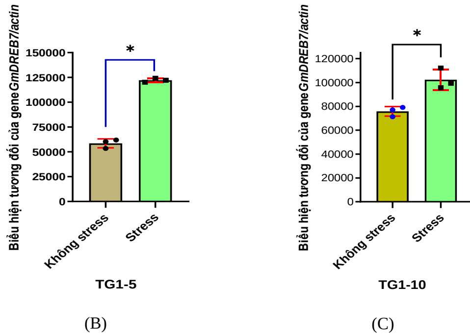
Hình 3.19. Biểu đồ so sánh mức độ phiên mã của gene GmDREB7 bằng phương pháp qRT-PCR ở các dòng đầu tương chuyển gene thể hệ TG1 và cây WT trong điều kiện không xử lý stress và xử lý stress mạn.
