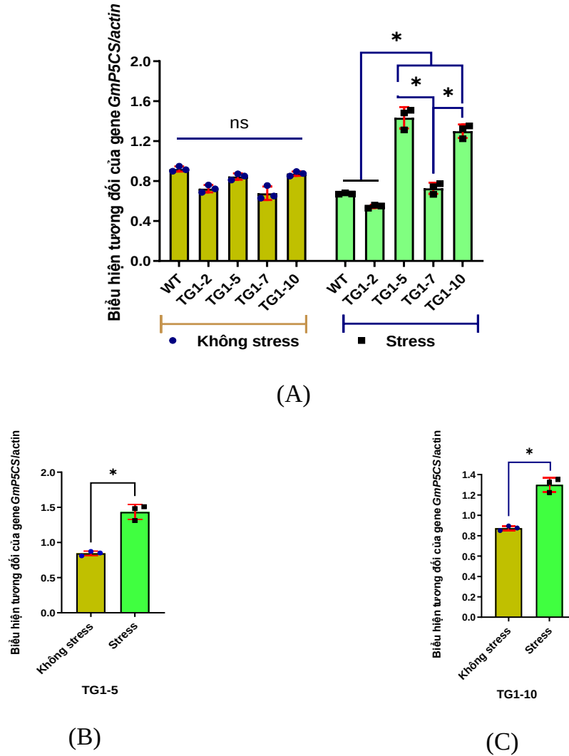
Hình 3.20. Biểu đồ so sánh mức độ phiên mã gene GmP5CS ở bốn dòng đậu tương chuyển gene thể hệ TG1 và cây WT bằng phương pháp qRT-PCR.
