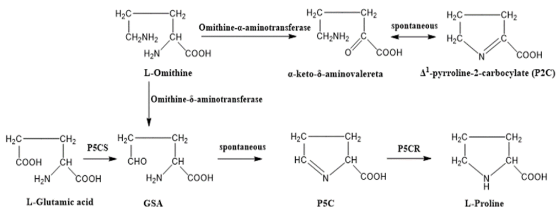
Hình 1.5. Con đường sinh tổng hợp proline ở thực vật bậc cao [31].
