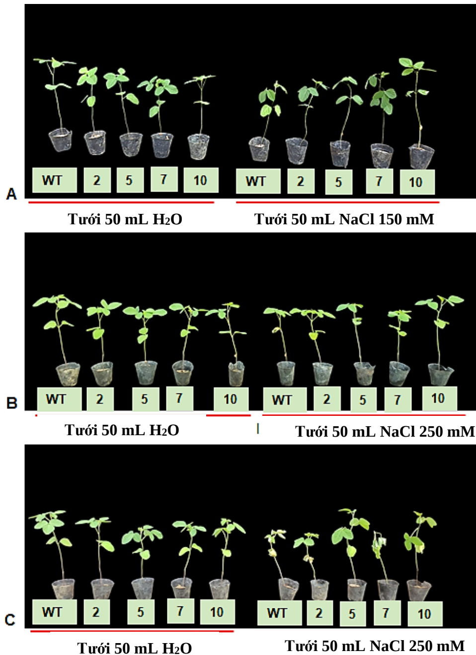
Hình 3.18. Hình ảnh cây đậu tương chuyển gene ở thể hệ TG1 và cây đối chứng trong điều kiện tưới nước và xử lý stress mặn.
