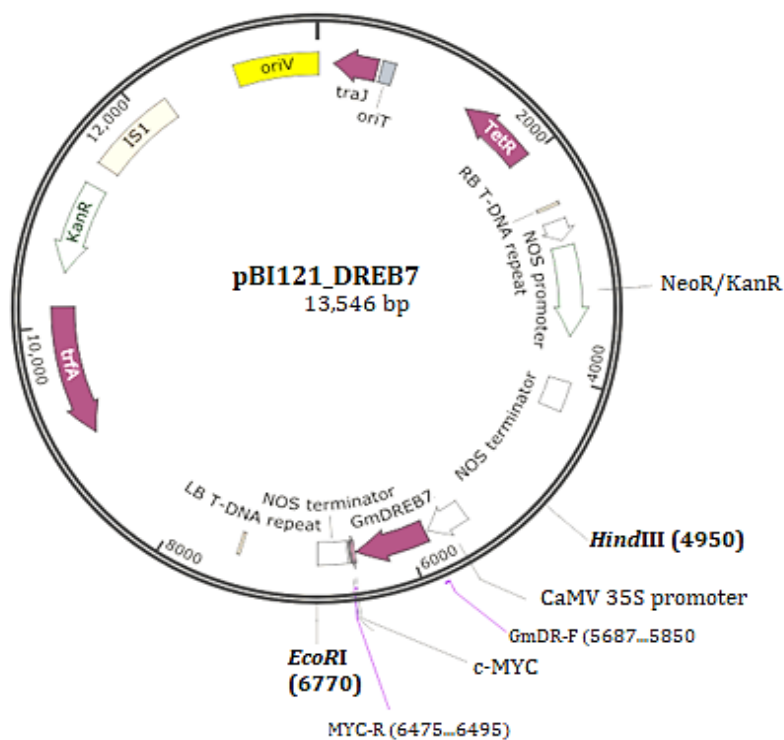
Hình 3.15. Sơ đồ cấu trúc vector pBI121_ GmDREB7 .
