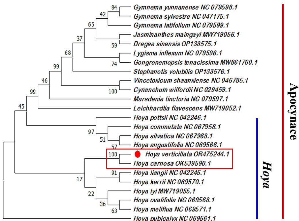
Hình 3.9. Sơ đồ phát sinh chủng loại sử dụng vùng đệm trnK-rps16 của hệ gene lục lạp H. verticillata var. verticillata và của các loài khác thuộc họ Apocynaceae
