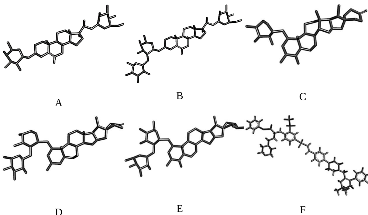
Hình 3.16. Cấu trúc 3D của các phân tử thử nghiệm. Các phân tử thử nghiệm gồm 05 saponin: (A) Hợp chất 1 ; (B) Hợp chất 2 ; (C) 3 \beta ,4 \alpha -dihydroxy-5 \beta -spirost-(25)27-en-1 \beta -yl O - \alpha -L-arabinopyranoside ( 3 ); (D) 3 \beta -hydroxy-5 \beta -spirost-25(27)-en-1 \beta -yl O - \alpha -L-rhamnopyranosyl-(1 \rightarrow 2)- \beta -D-xylopyranoside ( 4 ); (E) (23S,24S,25S)-3 \beta ,4 \alpha ,23,24-tetrahydroxy-5 \beta -spirostan-1 \beta -yl O - \alpha -L-rhamnopyranosyl-(1 \rightarrow 2)- \beta -D-fucopyranoside ( 5 ); và chất đối chứng là (F) Navitoclax.
